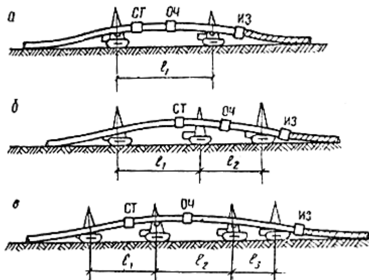
Рис. 12. Схемы расположения трубоукладчиков и машин в изоляционно-укладочной колонне для трубопроводов различных диаметров: а - 529- мм; б - 720-1020 мм; в - 1220-1420 мм; ОЧ - очистная машина; ИЗ - изоляционная машина; СТ - сушильная установка; l_1, l_2, l_3 - расстояния между трубоукладчиками
