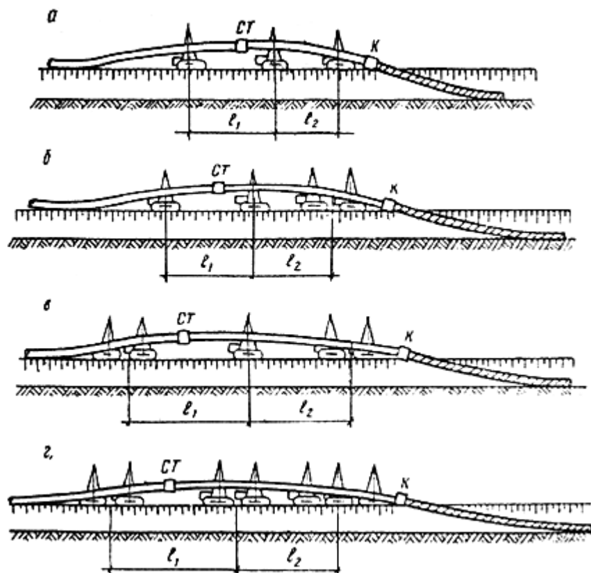
Рис. 10. Схемы расстановки трубоукладчиков и машин в изоляционно-укладочной колонне при совмещенном способе производства работ для трубопроводов различных диаметров: а - 529-820 мм; б - 1020 мм; в - 1220 мм; г - 1420 мм; СТ - сушильная установка; К - комбайн для очистки и изоляции трубопровода; l_1, l_2 - расстояния между трубоукладчиками и группами трубоукладчиков
