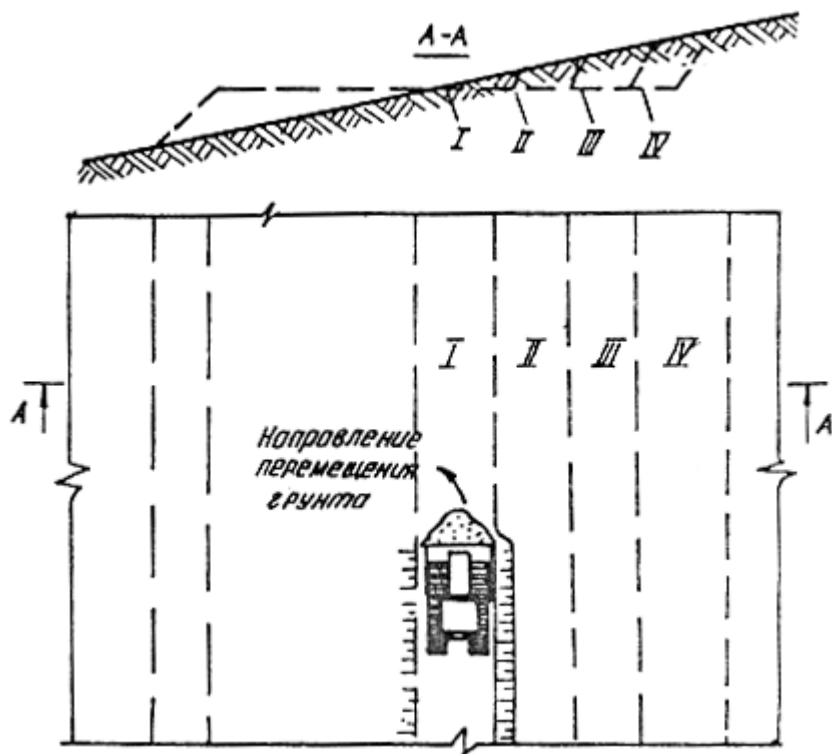
Рис. 3. Схема разработки полок на склонах продольными проходами бульдозера: I, II, III, IV - призмы разработанного грунта
