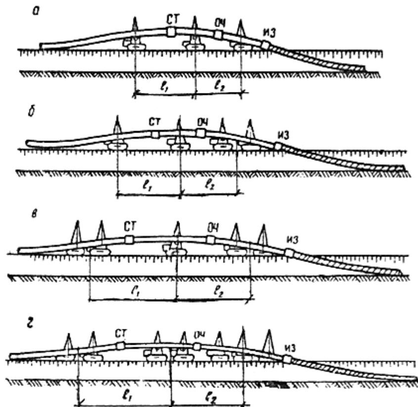
Рис. 9. Схемы расположения трубоукладчиков и машин в изоляционно-укладочной колонне при совмещенном способе производства работ для трубопроводов различных диаметров: а - 529-820 мм; б - 1020 мм; в - 1220 мм; г - 1420 мм; ОЧ - очистная машина; ИЗ - изоляционная машина; СТ - сушильная установка; l_1, l_2 - расстояния между трубоукладчиками и группами трубоукладчиков
