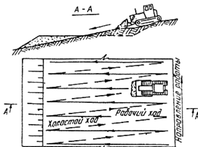
Рис. 2. Схема разработки полки на склонах поперечными проходами бульдозера
