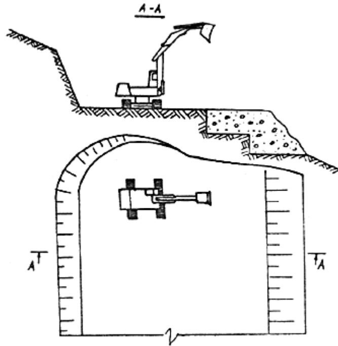
Рис. 4. Схема разработки полок экскаватором
