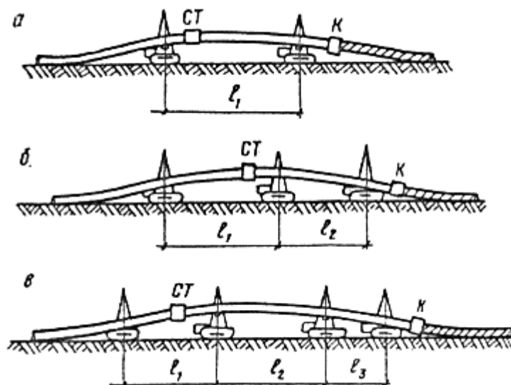
Рис. 11. Схемы расположения трубоукладчиков и машин в изоляционной колонне для трубопроводов различных диаметров: а - 529- мм; б - 720-1020 мм; в - 1220-1420 мм; СТ - сушильная установка; К - комбайн для очистки и изоляции трубопровода; l_1, l_2, l_3 - расстояния между трубоукладчиками
