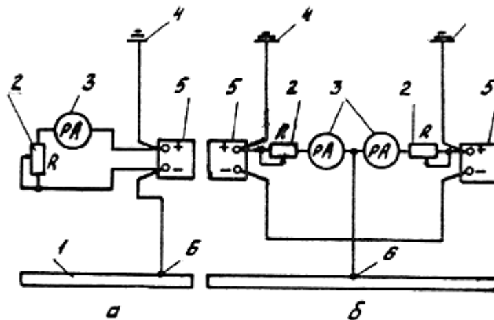
Рис. 32. Схема включения приборов и устройств при испытании преобразователей катодной защиты в режиме максимальной нагрузки: а - при работе одного преобразователя на один очаг анодного заземления; б - при работе двух преобразователей на два очага анодного заземления; 1 - трубопровод; 2 - регулируемый добавочный резистор нагрузки; 3 - амперметр; 4 - анодное заземление; 5 - преобразователь катодной защиты; 6 - точка дренажа
