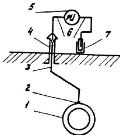
Рис. 31. Схема измерений разности потенциалов "труба - земля": 1 - трубопровод, 2 - контакт с трубопроводом; 3 - катодный вывод; 4 - контрольно-измерительный пункт; 5 - многопредельный вольтметр; 6 - измерительные провода; 7 - неполяризующийся медно-сульфатный электрод
