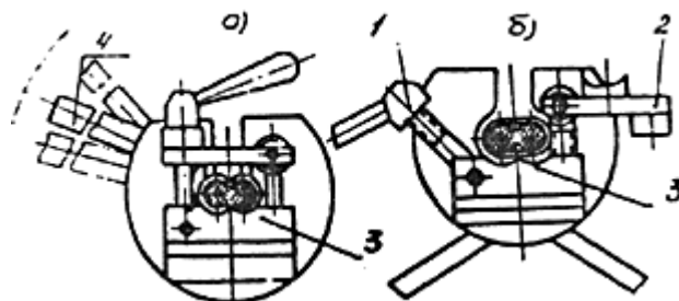
Рис. 6. Зажимные узлы приспособления МИ-189А:
