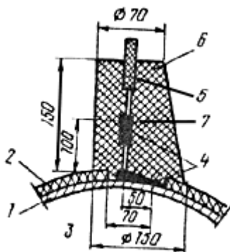
Рис. 20. Изолированное сварное соединение: 1 - трубопровод; 2 - изоляция трубопровода; 3 - Г-образный стальной стержень; 4 - сварные соединения; 5 - кабель; 6 - битумно-резиновая мастика; 7 - изоляционная лента
