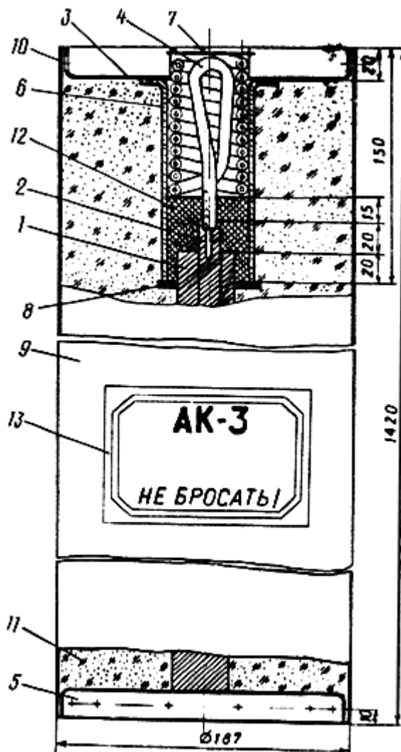
Рис. 3. Заземлитель анодный АК-3:
