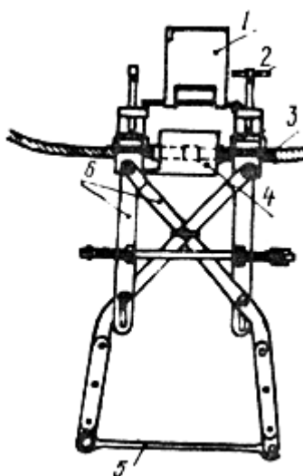
Рис.10. Сварочные клещи типа АТСП-50-185: 1 - защитный кожух; 2 - зажимное устройство; 3 - концы соединительных проводов, 4 - термитный патрон; 5 - крючок; 6 - рама пружины
