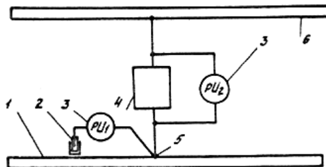
Рис. 33. Схема включения измерительных приборов при пусконаладочных работах на электродренажных установках: 1 - трубопровод; 2 - неполяризуемый медно-сульфатный электрод сравнения; 3 - вольтметр; 4 - электродренажная установка; 5 - точка дренажа; 6 - рельсовая сеть
