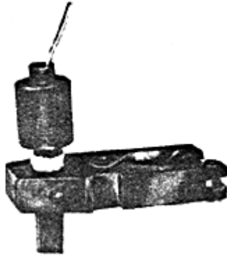
Рис. 17. Введение присадочного прутка из алюминиевой проволоки в кокиль термитного патрона марки АС при сварке алюминиевой жилы кабеля со стальным стержнем
