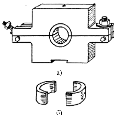
Рис. 23. Охладитель со сменными вкладышами: а - охладитель; б - сменные вкладыши
