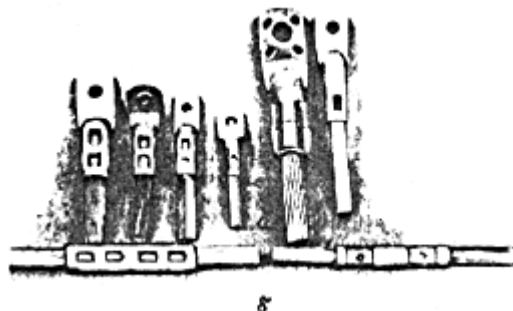
Рис. 27. Образцы оконцования алюминиевых жил кабелей, выполненные способом опрессовки:
