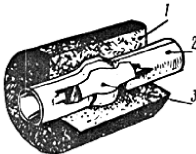
Рис .9. Термитный патрон марки АС для сварки жил проводов и кабелей: 1 - термитный патрон; 2 - кокиль; 3 - алюминиевый вкладыш
