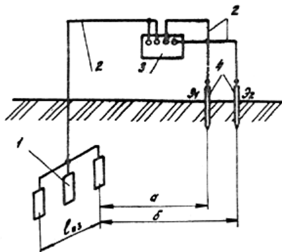
Рис. 30. Схема измерения сопротивления растеканию тока анодного заземления:
