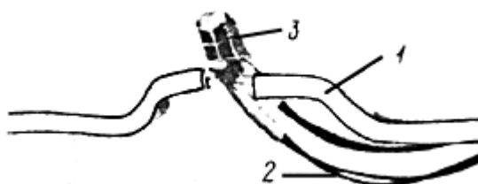
Рис. 29. Узел контактного соединения при монтаже анодных заземлителей:
